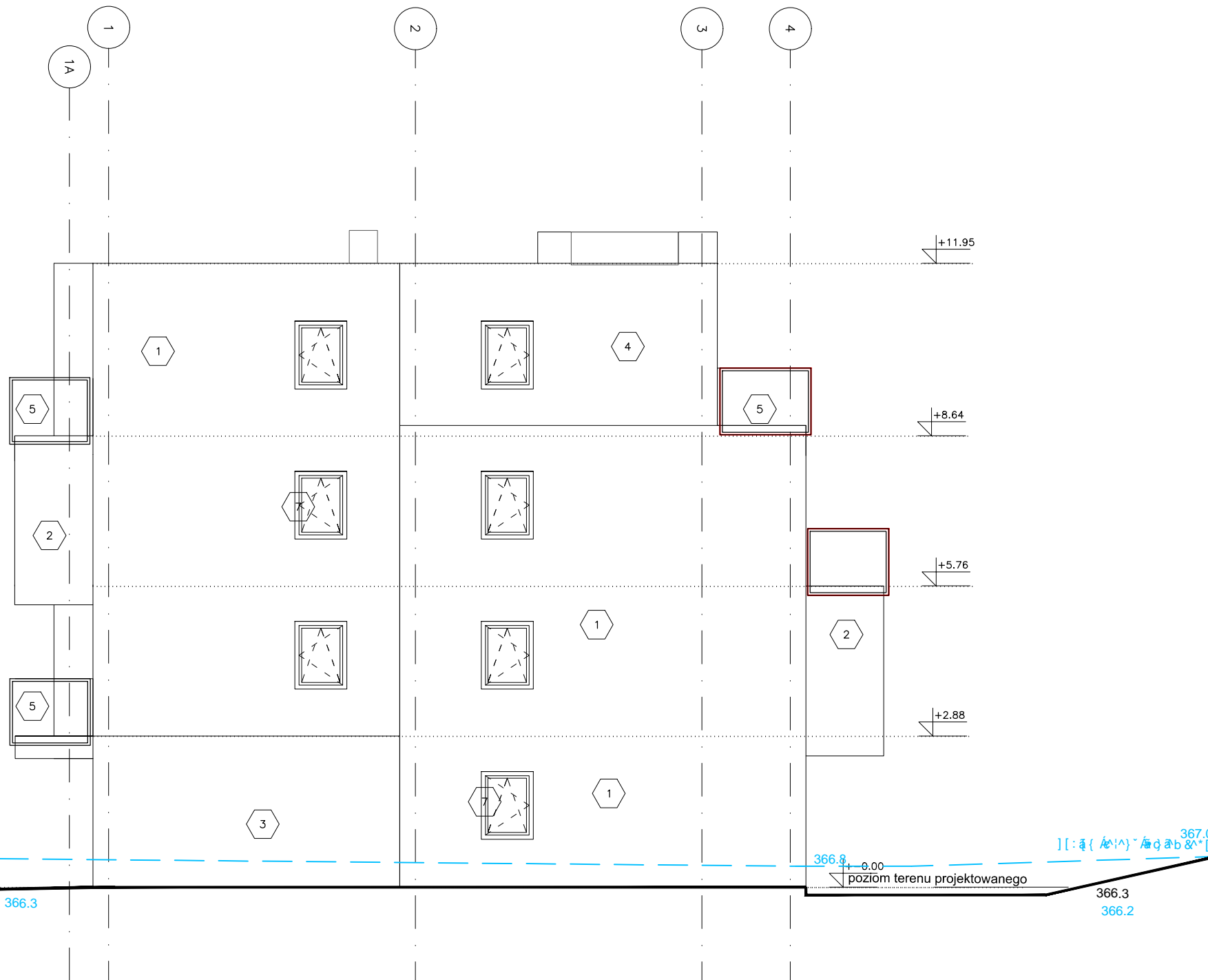
ELEWACJA PÓŁNOCNA
