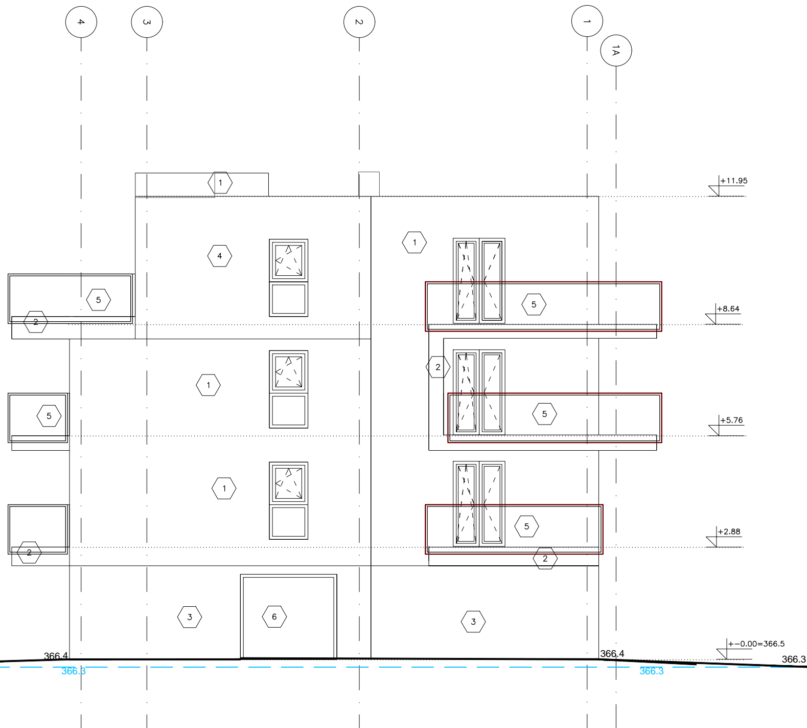
ELEWACJA POŁUDNIOWA
